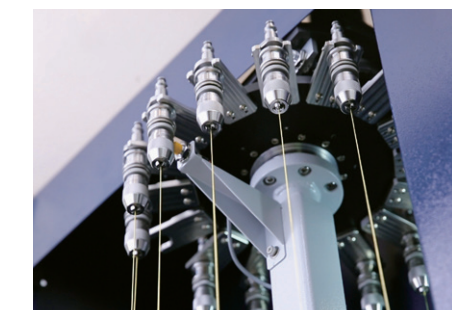
選配16電極銅管自動交換系統
